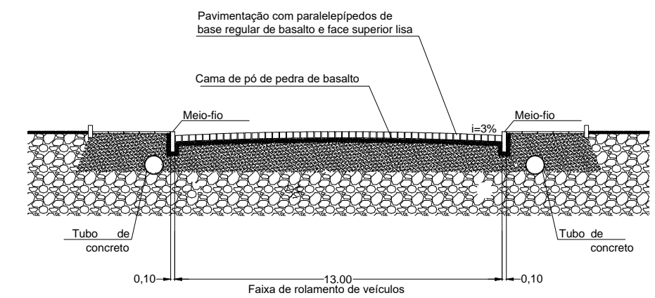
Perfil Transversal RUA "B" e "C"
