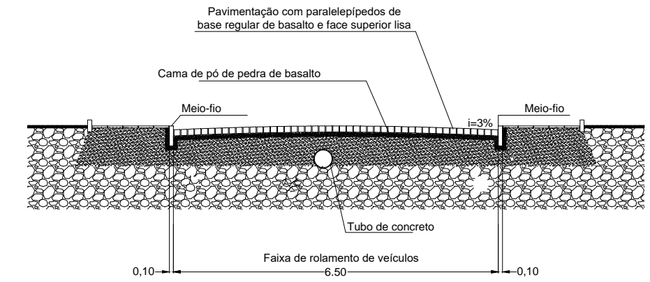
Perfil Transversal RUA "A"
